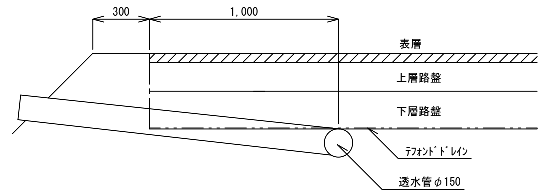
断面図 (樹無し) S=1/20
