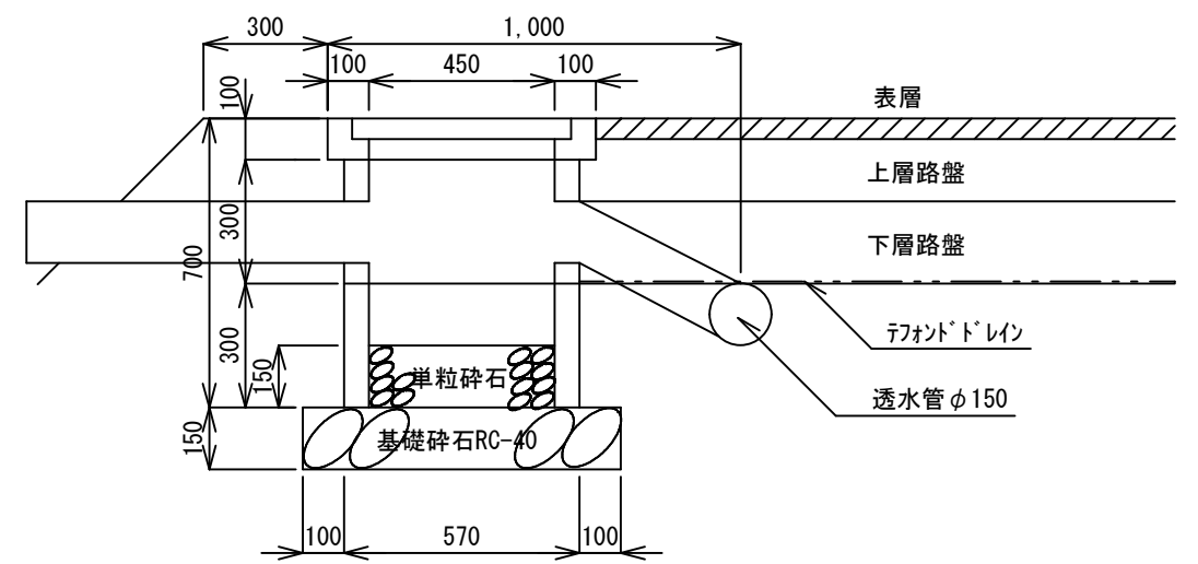
断面図 (樹無し) S=1/20
