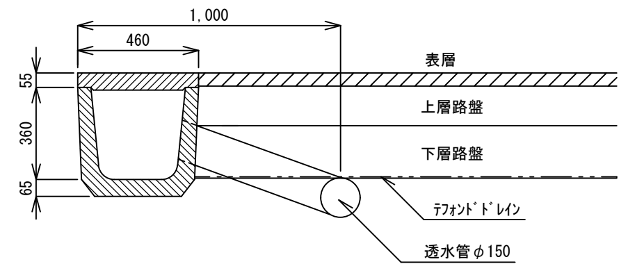
断面図 (樹無し) S=1/20
