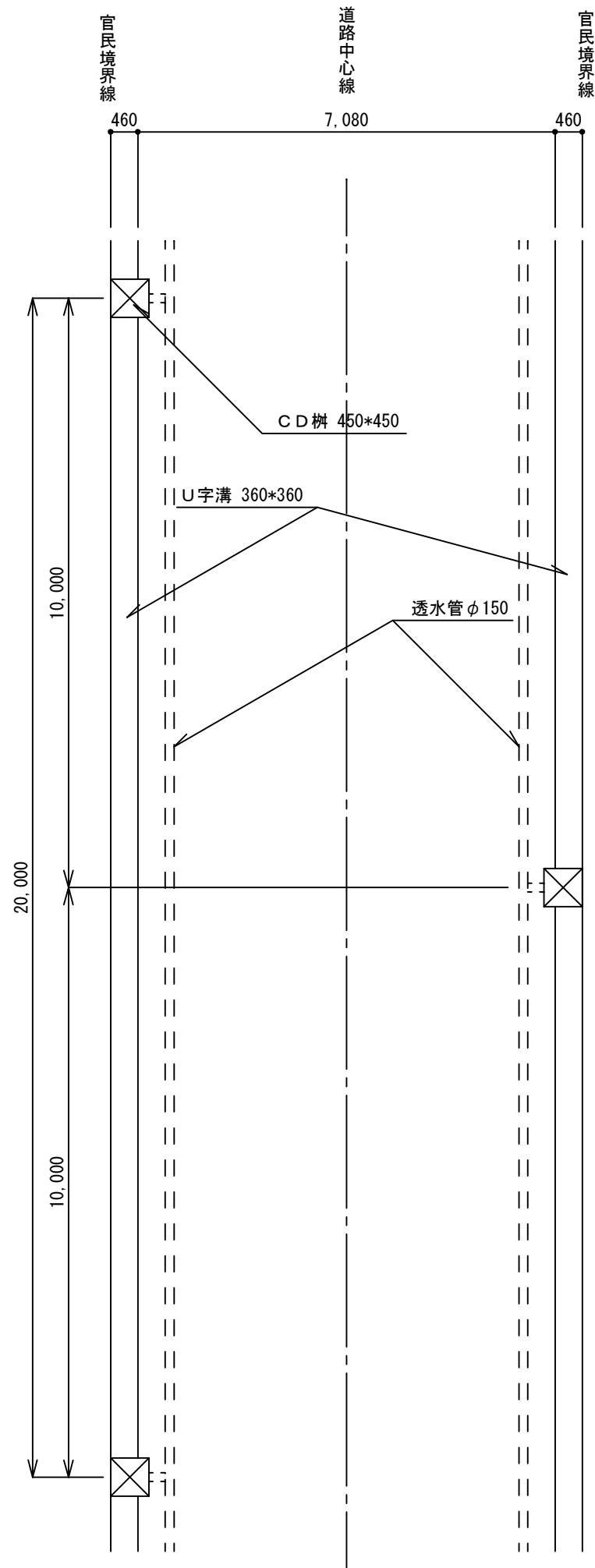
平面図 (樹使用) S=1/100
