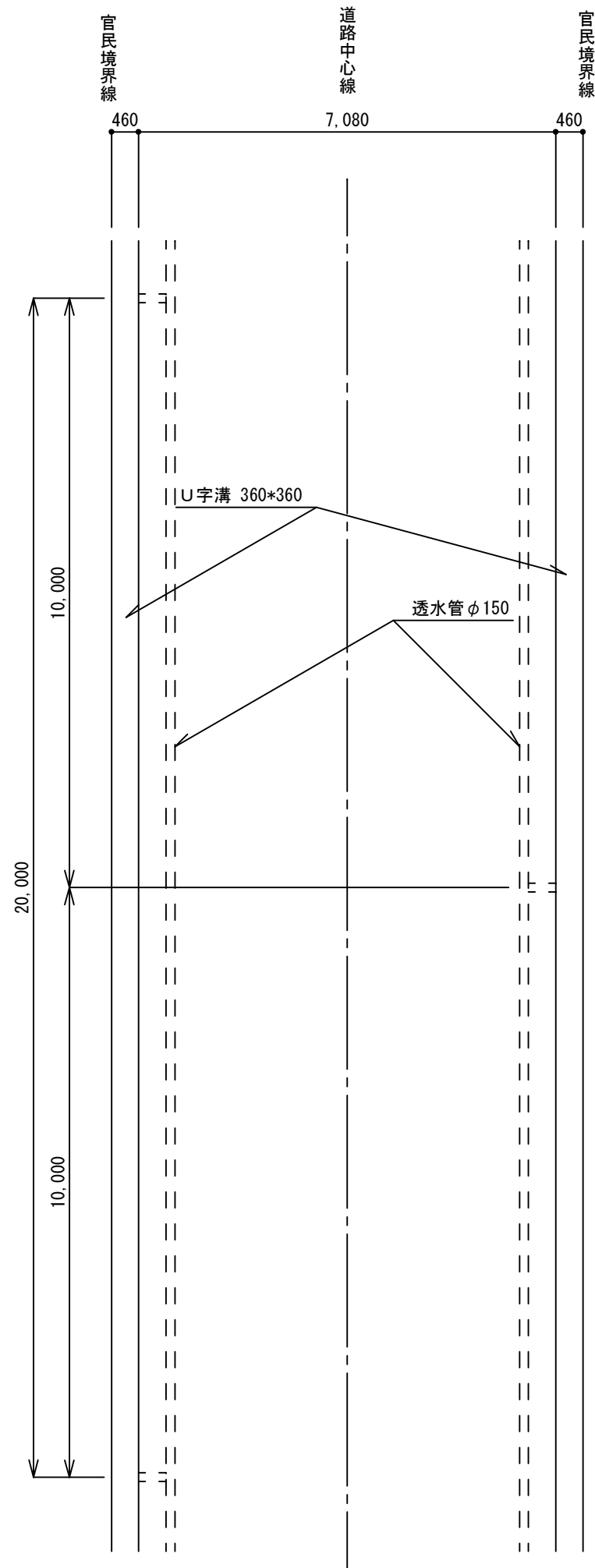
平面図 (樹無し) S=1/100
