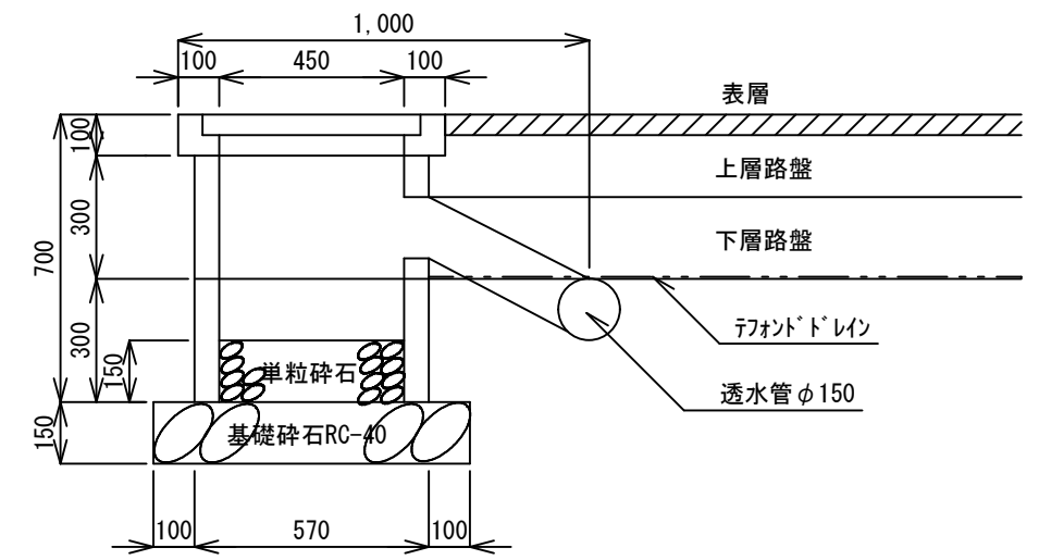
断面図 (樹無し) S=1/20
